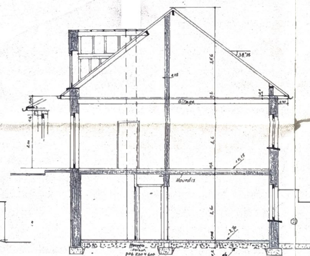
COUPE A-B
