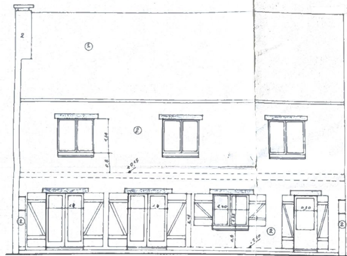
FAÇADE POSTERIEURE
