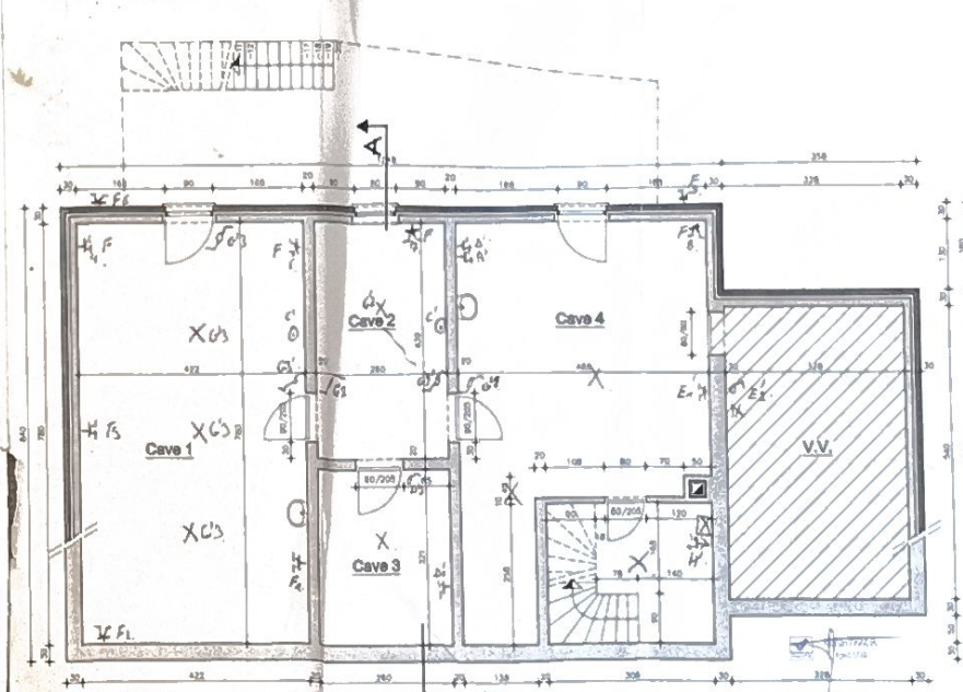
PLAN SOUS-SOL
