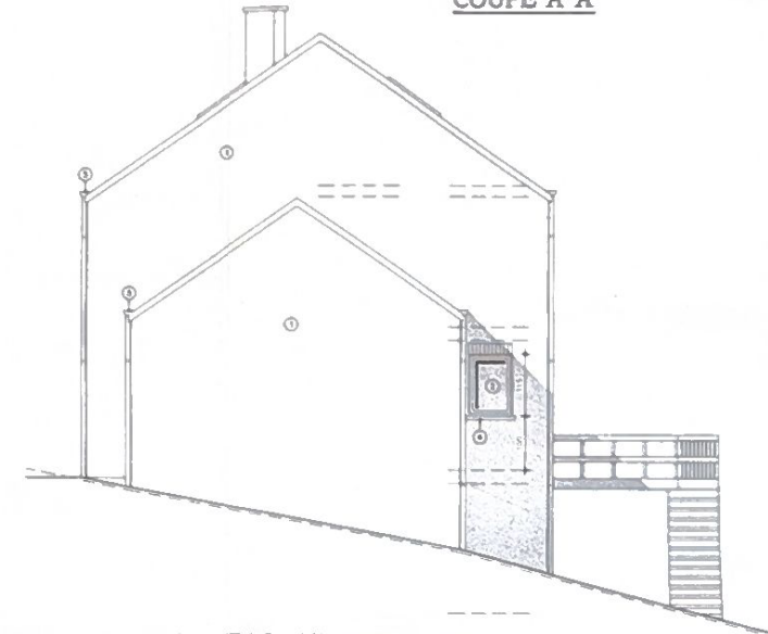
FACADE NORD-EST
