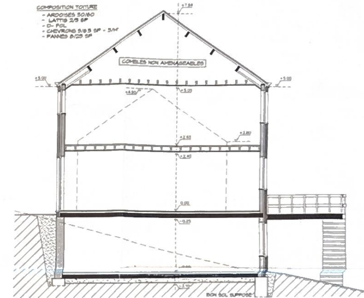
COUPE A-A
