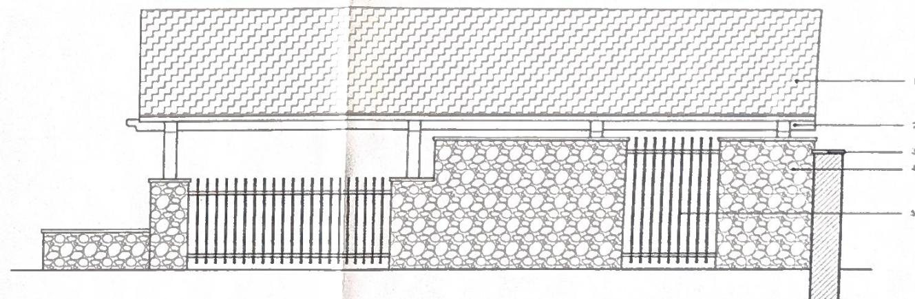
Facade Ouest
