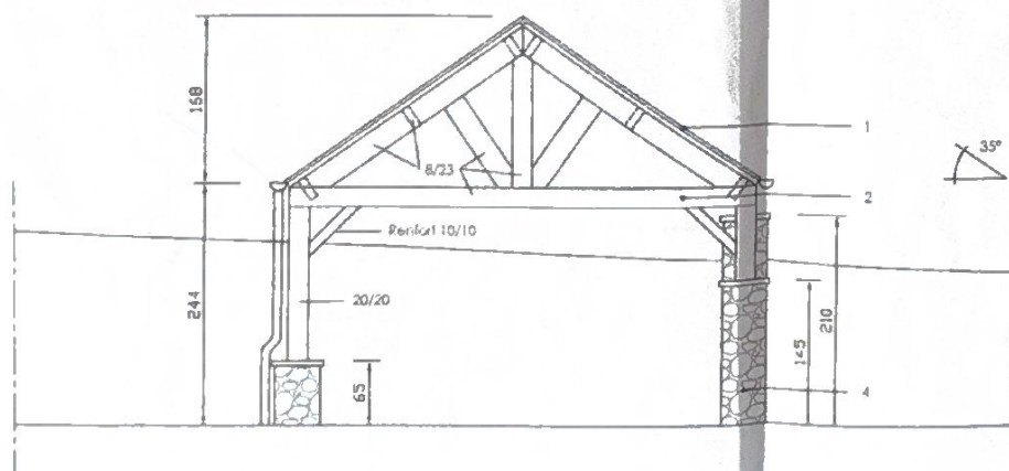
Facade Nord
